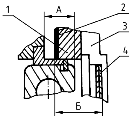
Рисунок 2- Регулировка осевого люфта вторичного вала.
